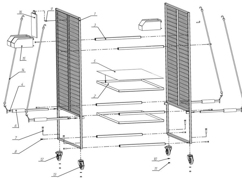
Рис.1 Схема сборки тележки
